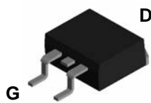
TO-263AB FDB Series
