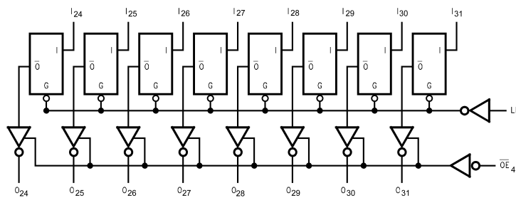
Byte 4 (24:31)
