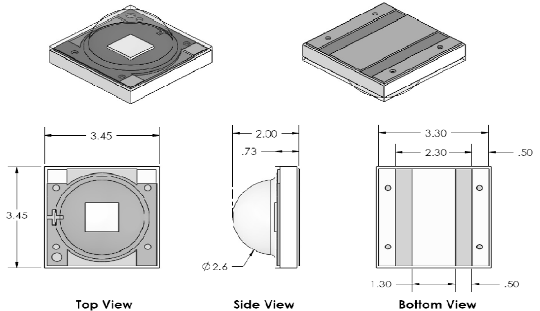
XPC / XPE / XPG XLamp
