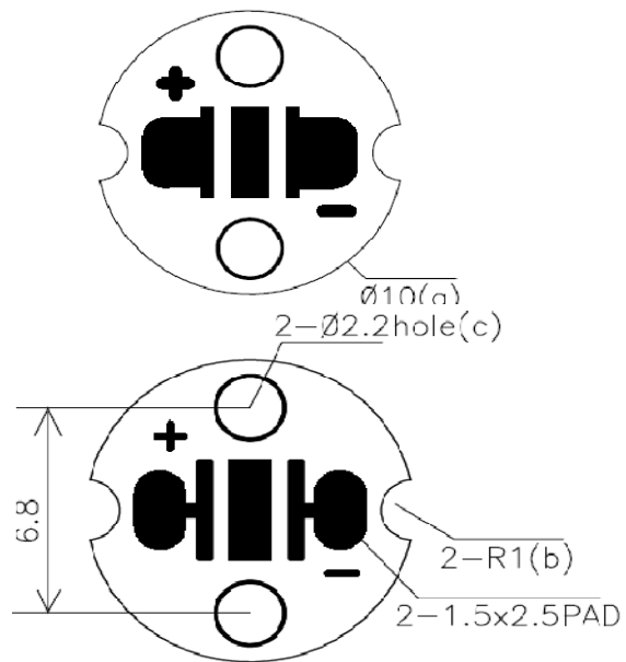
LBB2 MCPCB
