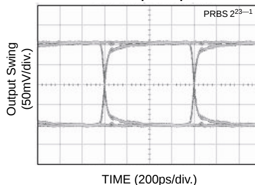
1.25Gbps Output
