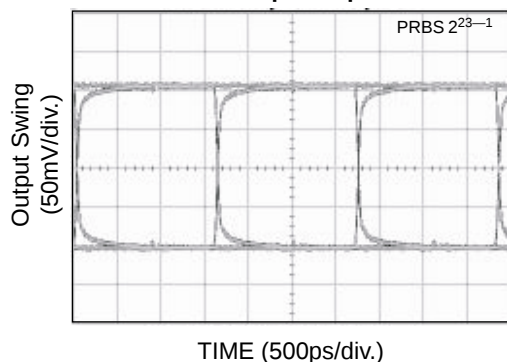
622Mbps Output
