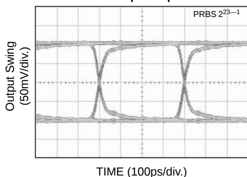
2.5Gbps Output
