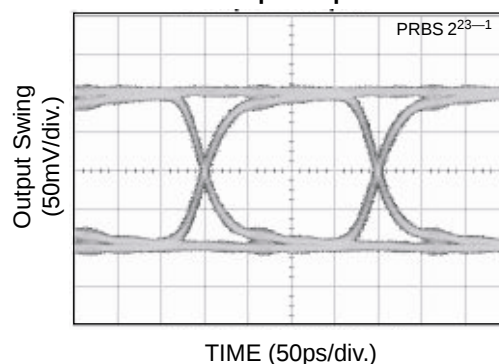
5Gbps Output
