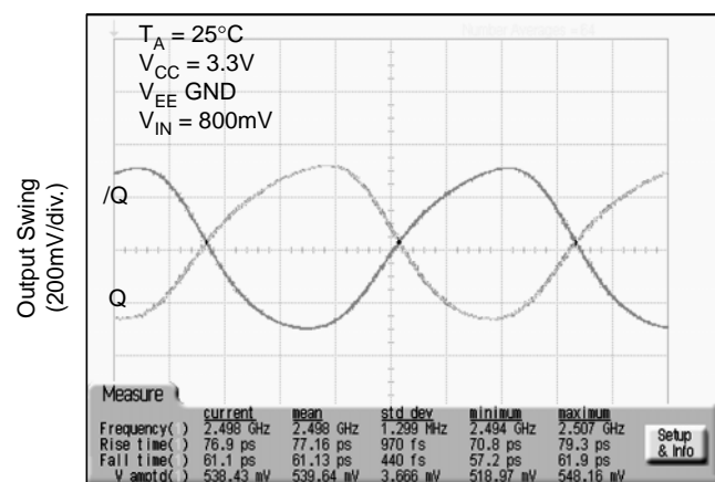
2.5GHz Output
