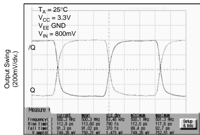
500MHz Output
