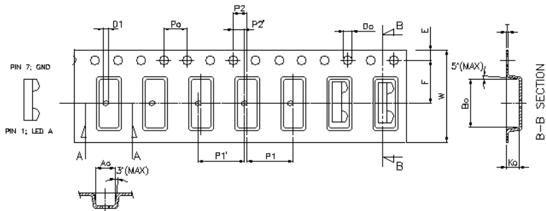
A-A SECTION
