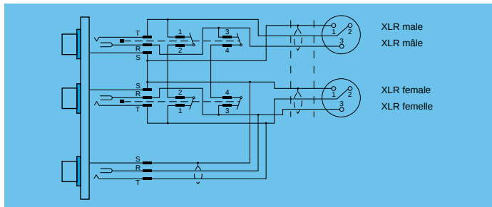
Front side connection Connexion avant
