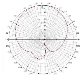
SAH35-90-16 Azimuth
