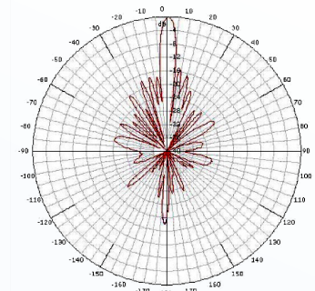
SAH35-90-16 E-Plane
