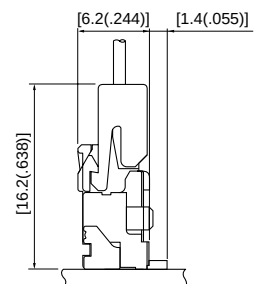
PAF Receptacle + PA Header
