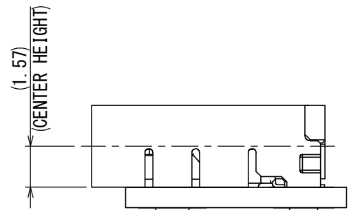
MOUNTING CONDITION (REF.) 実装状態図 (参考)
