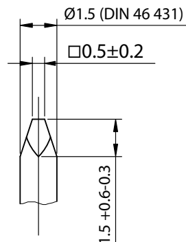
Detail Y M 5:1
