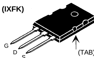
ISOPLUS 247™ (IXFR) E153432
