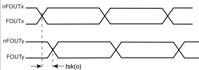
OUTPUT SKEW
