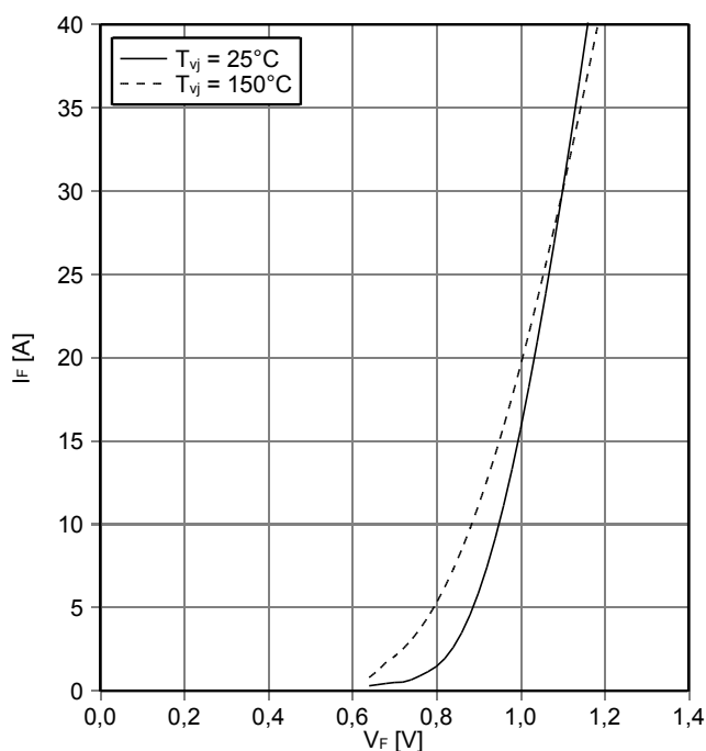
Durchlasskennlinie der Verpolschutz Diode B (typisch) forward characteristic of Inverse-polarity protection diode B (typical)
