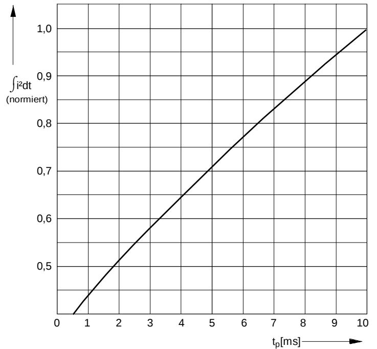
Bild / Fig. 2 Normiertes Grenzlastintegral / Normalized i^2t \int i^2 dt = f(t_p)
