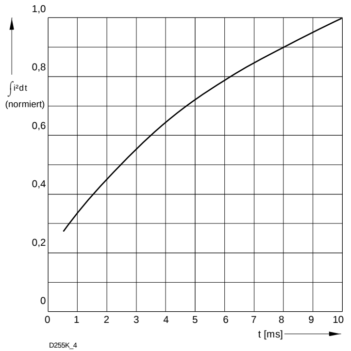
Bild / Fig. 2 Normiertes Grenzlastintegral / Normalized i^2 t \int i^2 dt = f(t_b)
