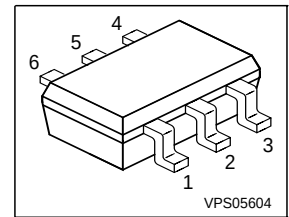
SOT-363
