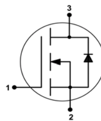
PG-SOT23
