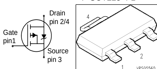
P-SOT223-4-1
