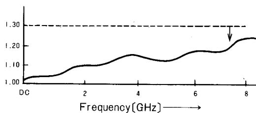
V.S.W.R.
