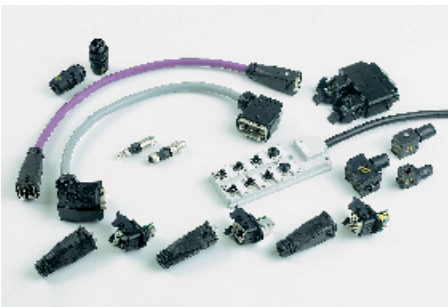
Feldbus- und Sensor-/Aktorkomponenten, Han-InduNet®-Systemkabel
