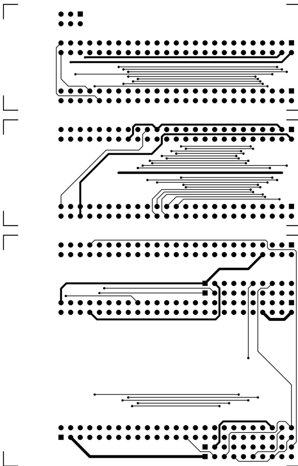
Top Layer
