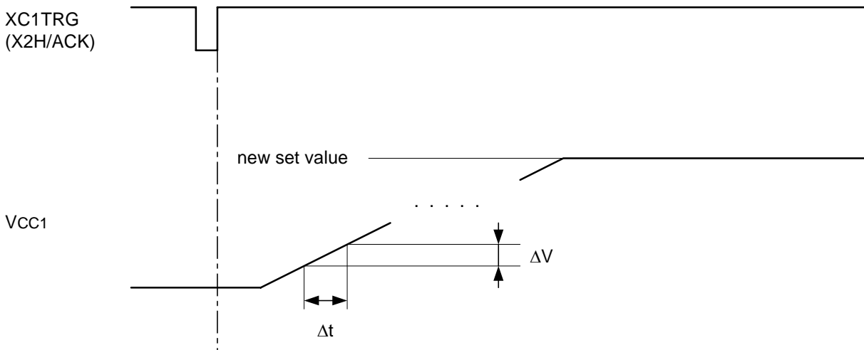
Fig.1 DVM function
