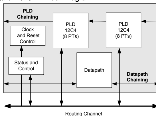
Figure 7-6. UDB Block Diagram
