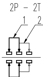
示意图 SCHEMATIC
