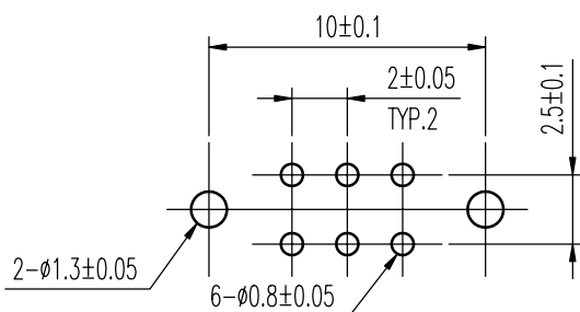
安装孔 PIERCING PLAN
