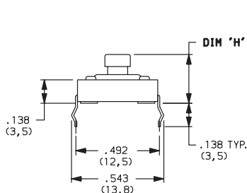
PTS125SJM73 SPST
