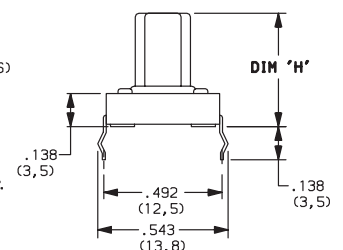
PTS125SM12 SPST
