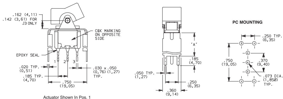
7101J1_BE2 SPDT
