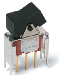
7101J1_BE2 SPDT
