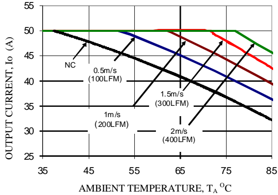
V_o=0.7V , V_{in}=12V
