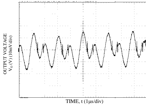
Vo=1.2V, Ta=25°C, Vin=12V, Io = Io,max
