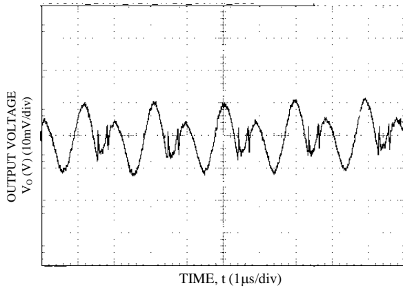
Vo=0.7V, Ta=25°C, Vin=12V, Io = Io,max
