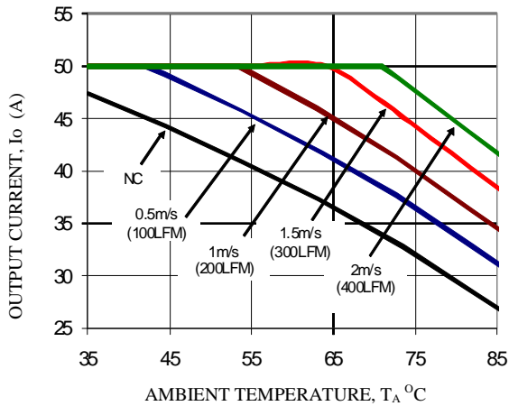
V_o=1.8V , V_{in}=12V
