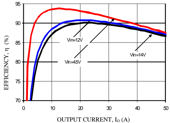
V_o=1.2V , T_a=25^\circ C
