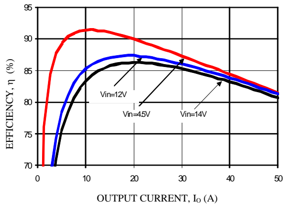
V_o=0.7V , T_a=25^\circ C
