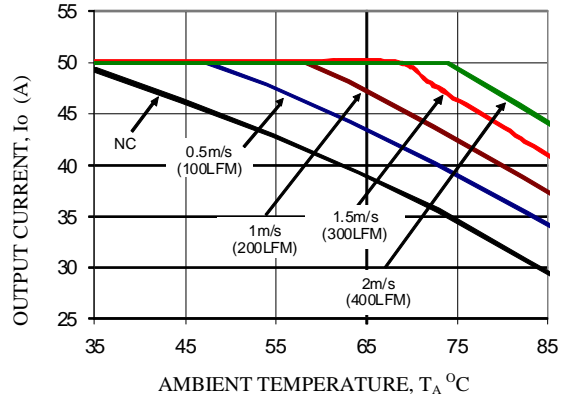
V_o=1.2V , V_{in}=12V
