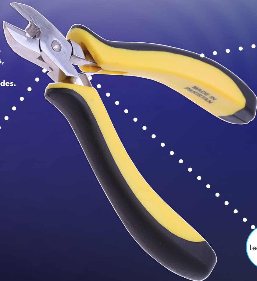
Tungsten Carbide Blades 79-80 HRC
