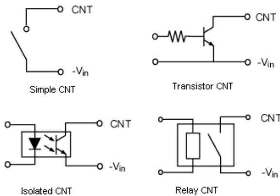
Fig. 51 CNT Circuit
