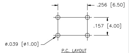
P.C. LAYOUT
