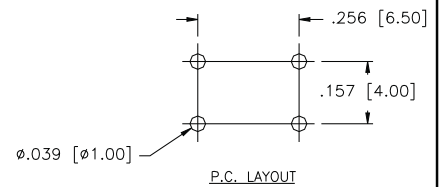
P.C. LAYOUT
