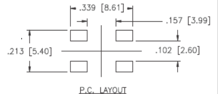
P.C. LAYOUT
