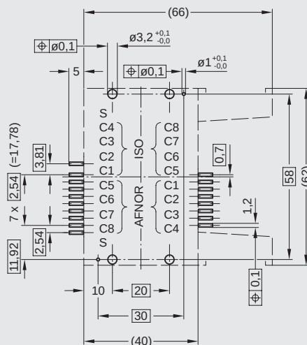
BESTÜCKUNGSSEITE / COMPONENTS SIDE
