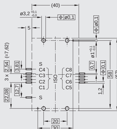
BESTÜCKUNGSSEITE / COMPONENTS SIDE
