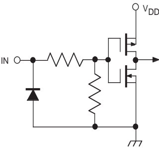
Dwg. EP-010-12
