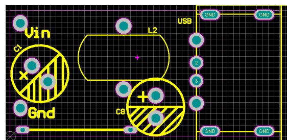
Top overlay
