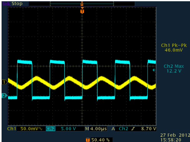
Vin=12V Io=1A
